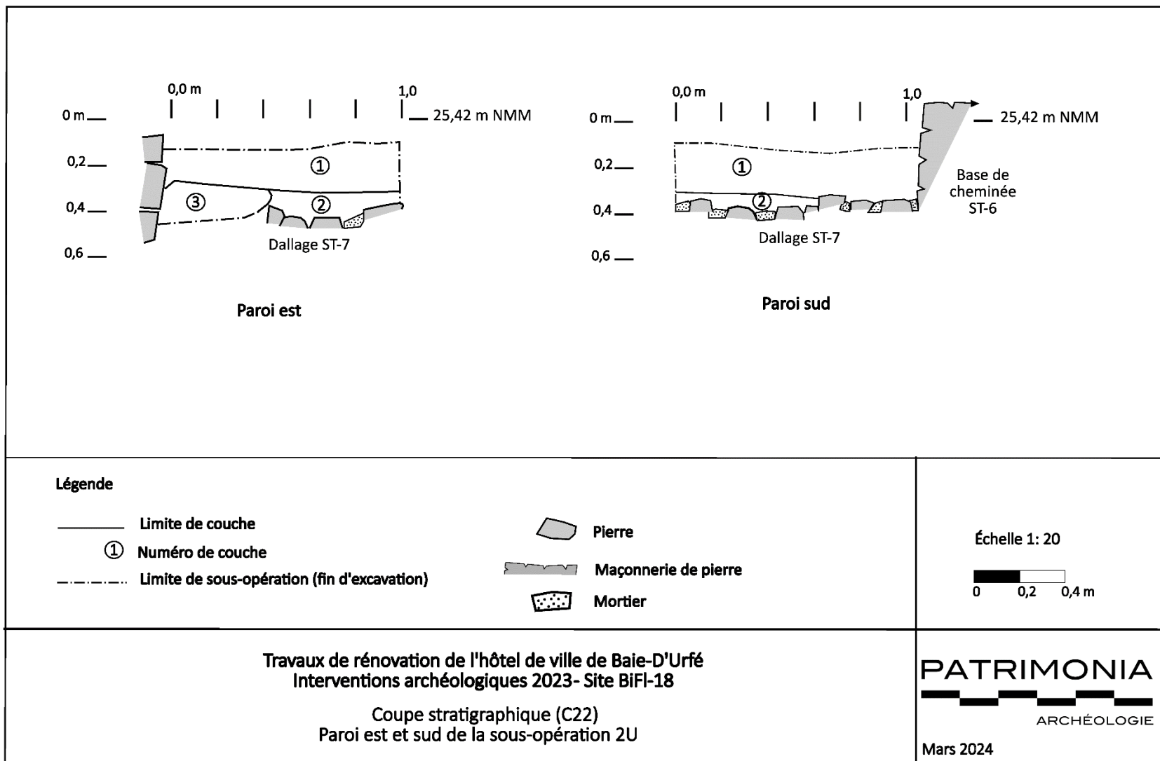
Figure 22. Coupe stratigraphique C22, paroi est et sud de la sous-opération 2U
