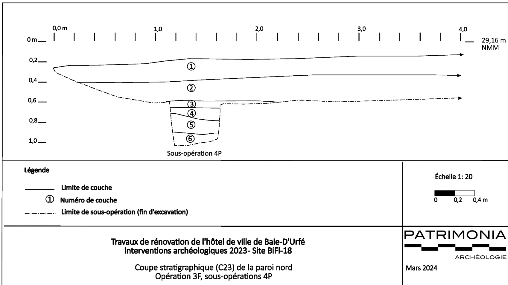
Figure 23. Coupe stratigraphique C23, paroi nord de l'opération 3F et sondage 4P
