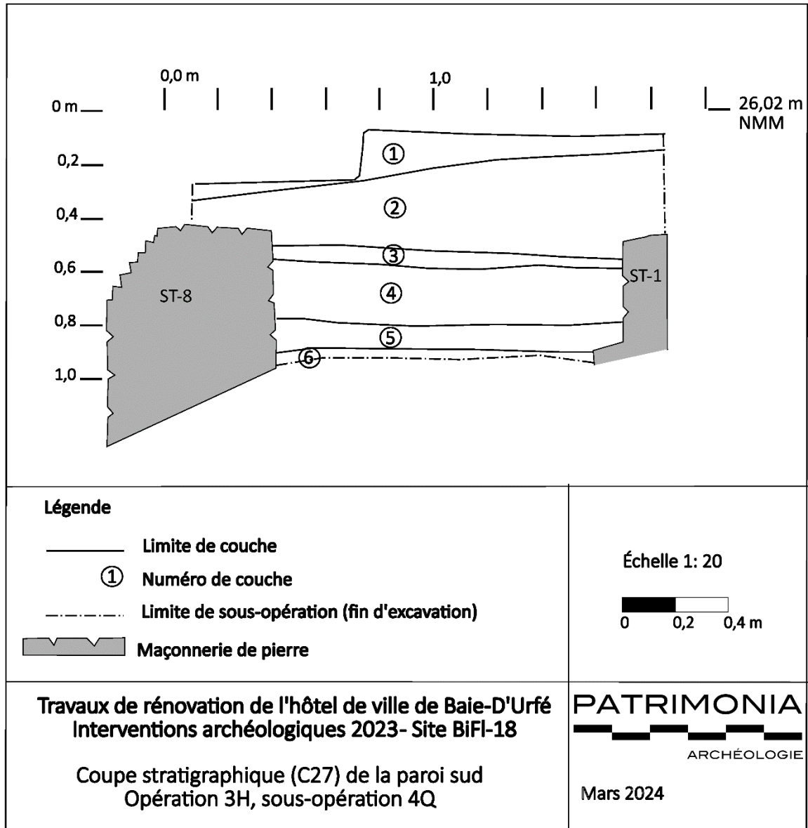
Figure 25. Coupe stratigraphique C27, paroi sud de l'opération 3H et sondage 4Q
