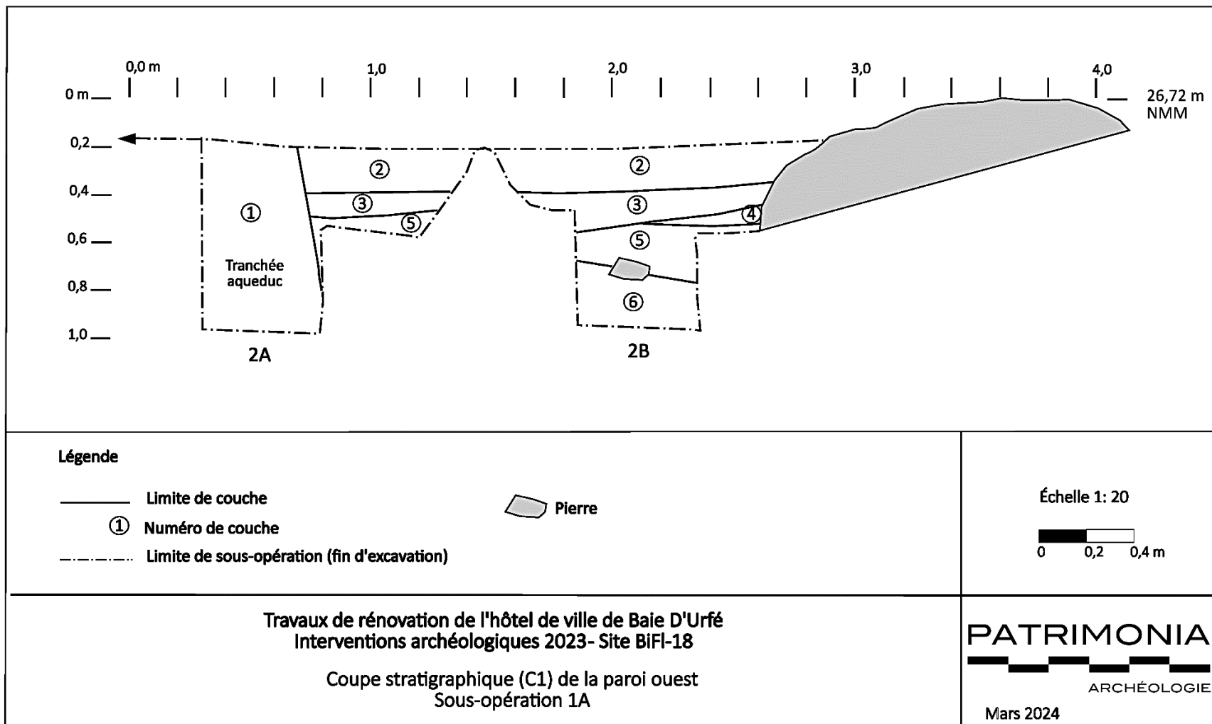
Figure 16. Coupe stratigraphique C1, paroi ouest de la sous-opération 1A et des sondages 2A et 2B
