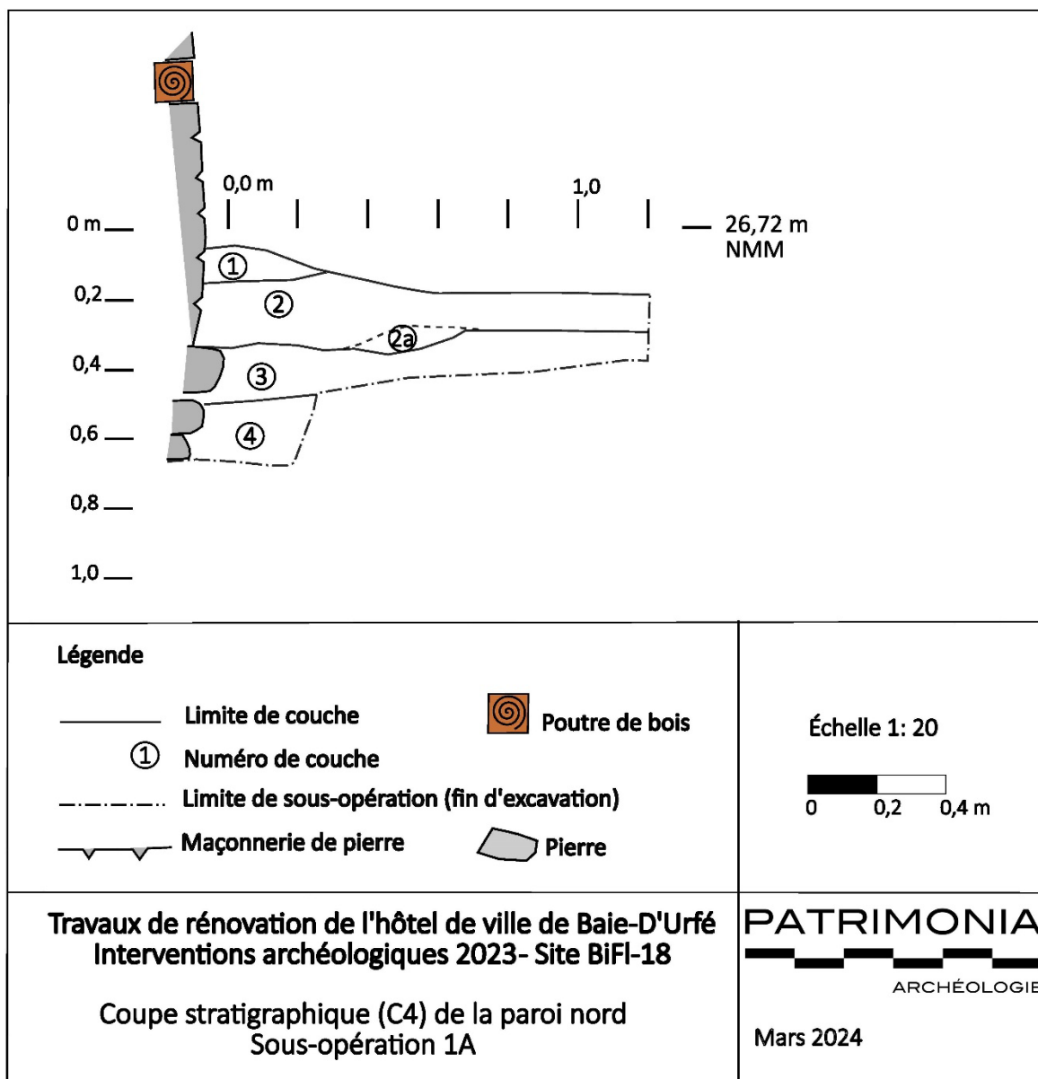
Figure 17. Coupe stratigraphique C4, paroi nord de la sous-opération 1A
