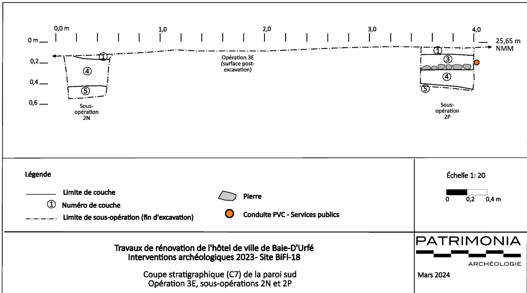
Figure 19. Coupe stratigraphique C7, paroi sud de l'opération 3E et des sondages 2N et 2P
