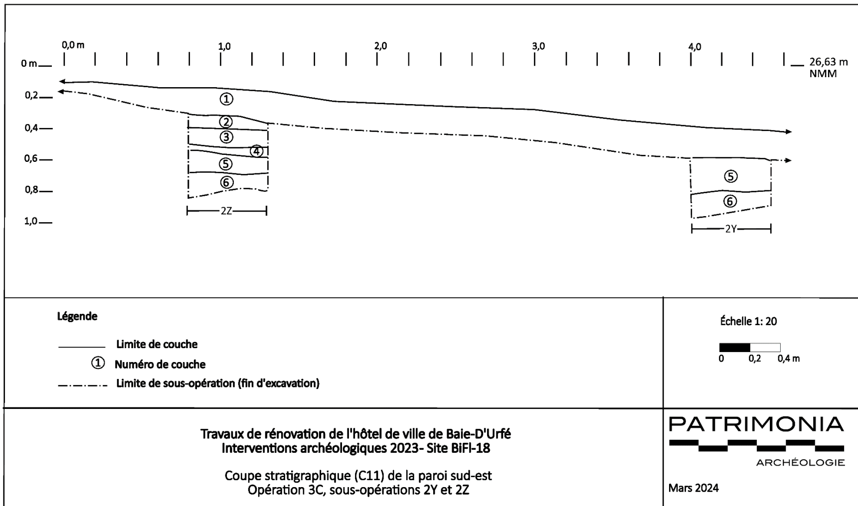
Figure 21. Coupe stratigraphique C11, paroi sud-est de l'opération 3C, sondages 2Y et 2Z
