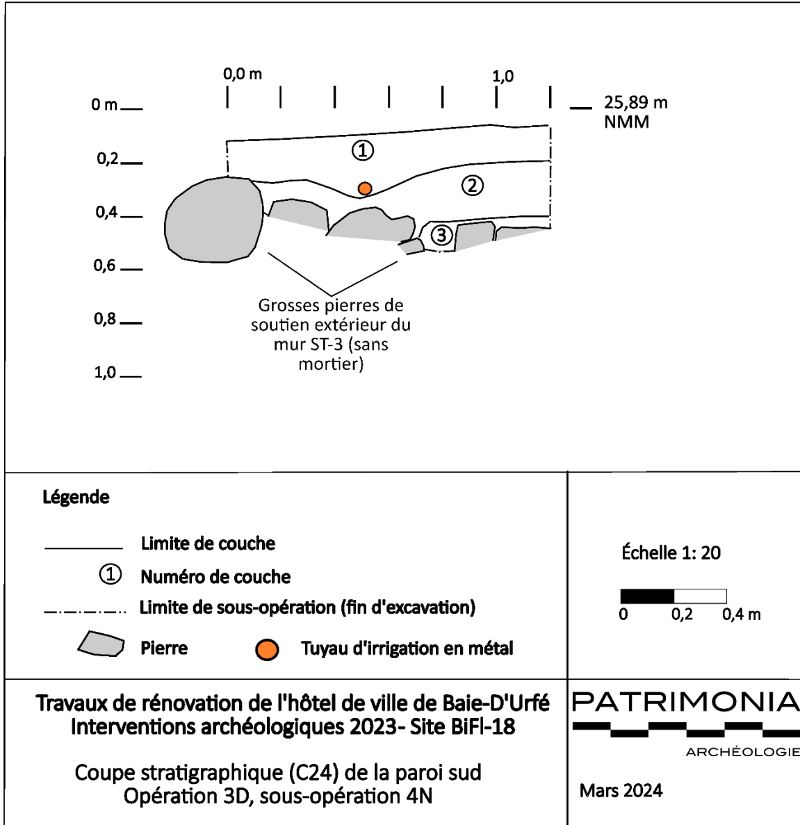
Figure 24. Coupe stratigraphique C24, paroi sud de l'opération 3D et sondage 4N
